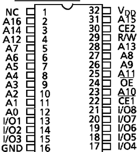
○ 32 PIN SOP
