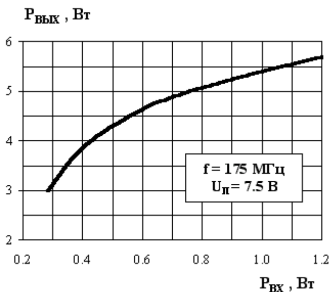
Зависимость выходной мощности от входной мощности
