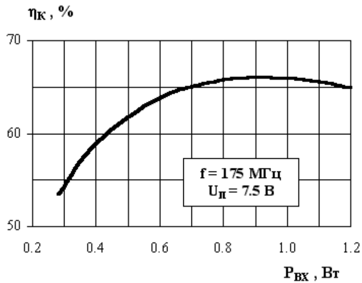
Зависимость коэффициента полезного действия коллектора от входной мощности
