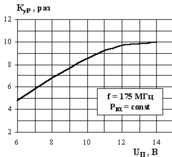
Зависимость коэффициента усиления по мощности
