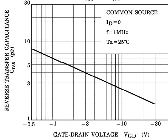
Crss - VGD
