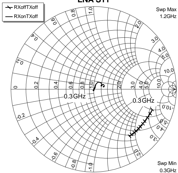
LNA S11
