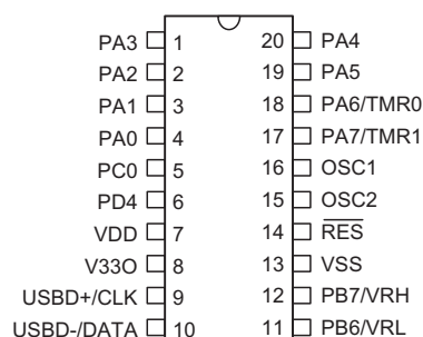
HT82K96E -20 SOP-A
