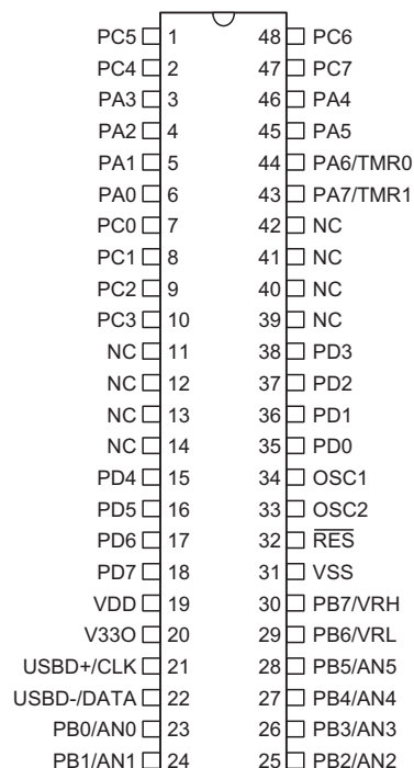
HT82K96E -48 SSOP-A
