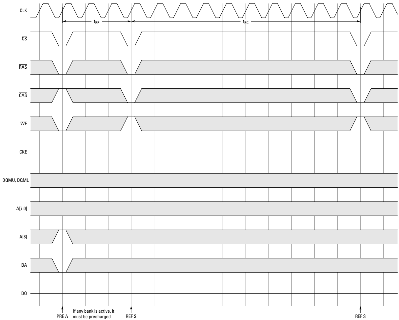
Figure 34. Auto-Refresh
