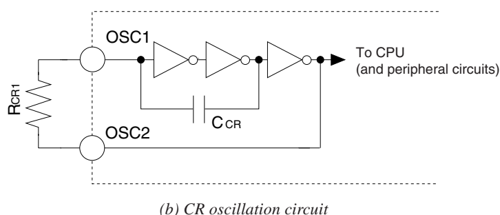
Fig. 4.4.2.1 OSC1 oscillation circuit
