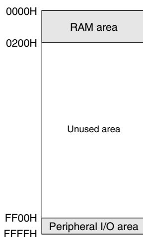
Fig. 4.1.1 Memory map
