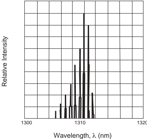
LONGITUDINAL MODE
