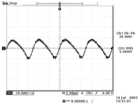
V_{in}=5 V, V_o=0.9 V
