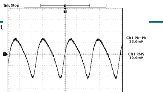
V_{in}=12 V, V_o=1.5 V
