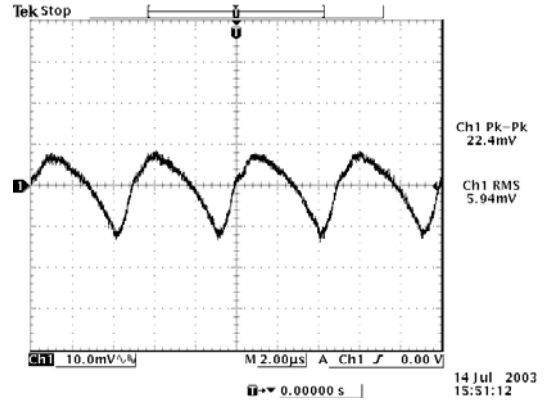
V_{in}=12 V, V_o=0.9 V
