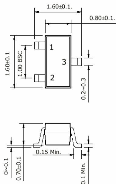
SOT - 523 unit : mm
