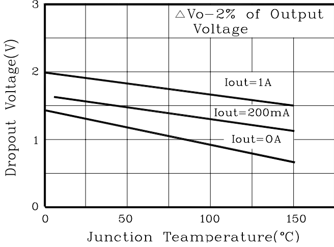
Fig. 1 V_{DVSE} vs T_j
