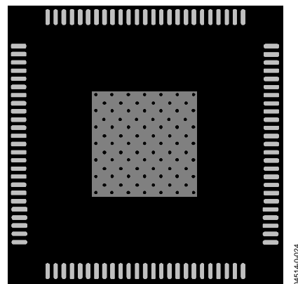
Figure 24. Solder Mask—Top Layer
